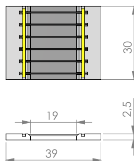
M1930E20 – Actuator Module only
